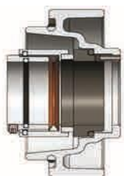
Kapseloitu mekaaninentiiviste
