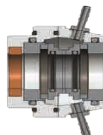
Kaksois-mekaaninentiiviste
